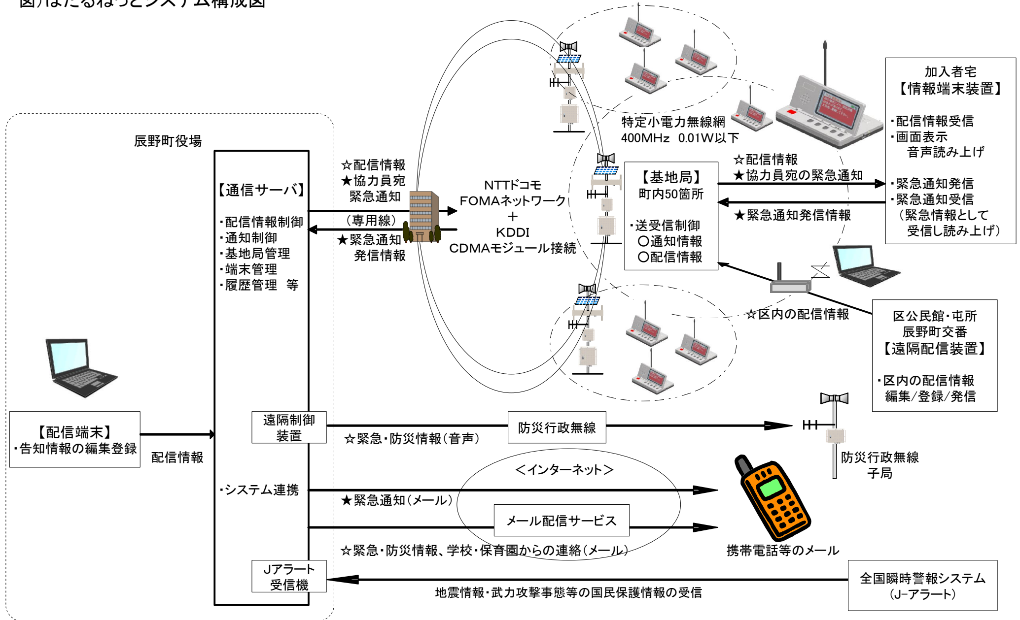
図) ほたるねっとシステム構成図
